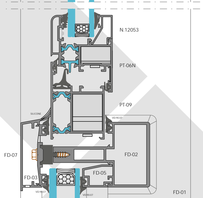
CORTE 10
