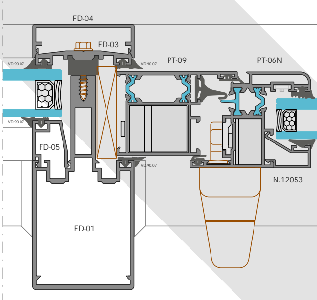
CORTE 11
