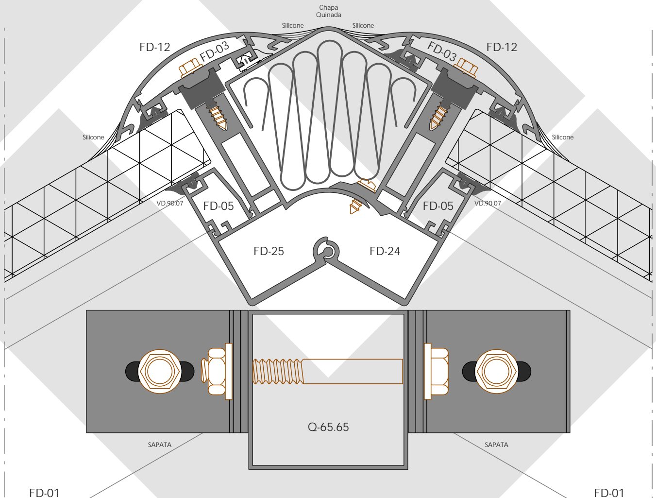
CORTE 18
