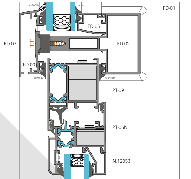
CORTE 9
